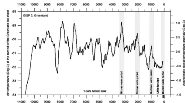
Bild 1. Temperaturkurva baserad på borrhärdar i Grönland. Som vi ser har temperaturen varierat över tid. Här är några historiskt belagda värmeperioder markerade (den minoiska värmeperioden, den romerska, den medeltida samt den moderna). Extra intressant är värmeperioden för 1 000 år sedan, då det var möjligt för vikingarna att skörda säd i Grönland. Det kan man ju inte idag.
